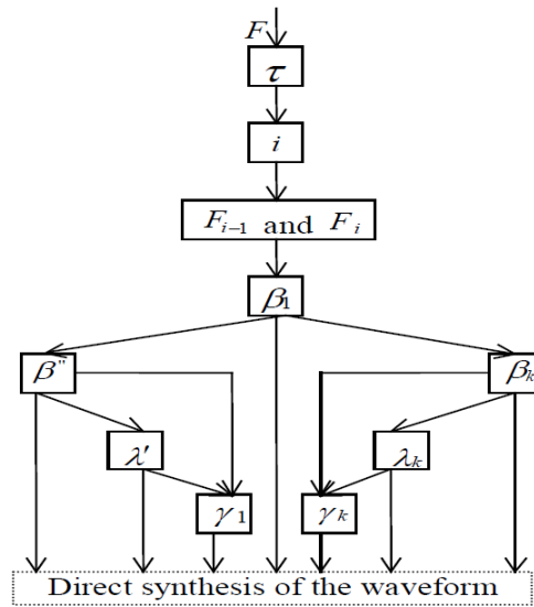
Рис. 2. Обобщенный алгоритм вычисления параметров сигналов управления инверторов с синхронной векторной ШИМ 2 .
