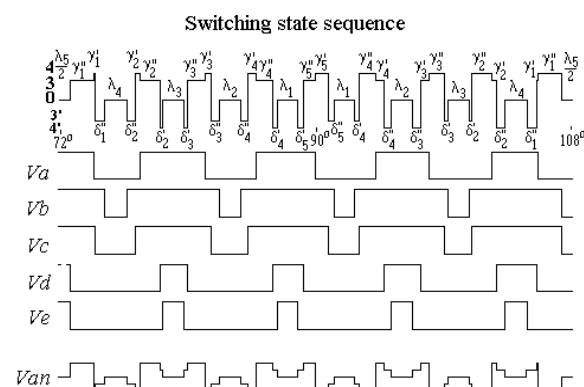
Рис. 20. Диаграмма состояния ключей и базовые напряжения пятифазного инвертора с в третьем секторе управления ( F = 31 \text{ Гц} ) 20 .
