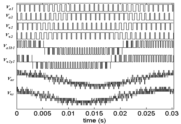
Рис. 24. Полярные напряжения V_{a1}, V_{a2} и V_{x1}, V_{x2} , линейные напряжения V_{a1b1} и V_{x1y1} , и фазные напряжения V_{as} и V_{xs} в шестифазной системе с непрерывной синхронной ШИМ 24 .
