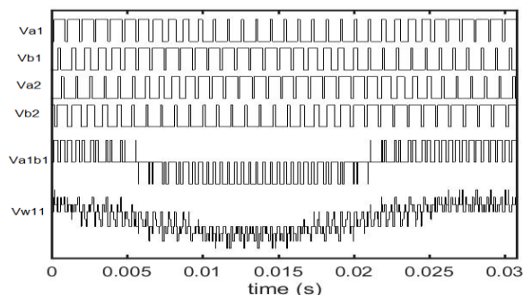
Рис. 8. Базовые напряжения в системе с синхронной непрерывной ШИМ 8 .
