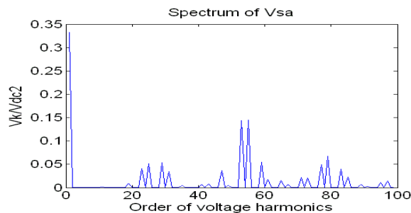
Рис. 13. Спектральный состав напряжения V_{sa} на рис. 12 13 .
